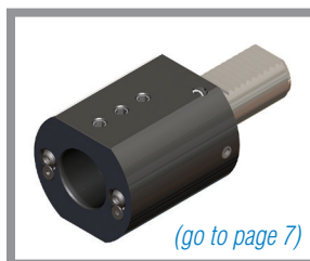
Part #: VDI30-ER32Z-E4 ER E4 DIN 6499
